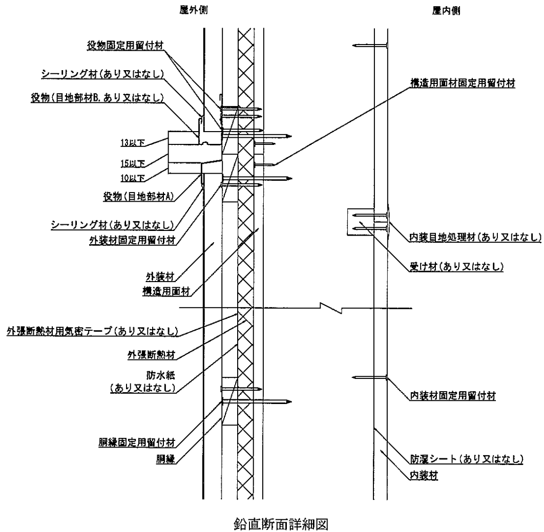
図 2 構造説明図
