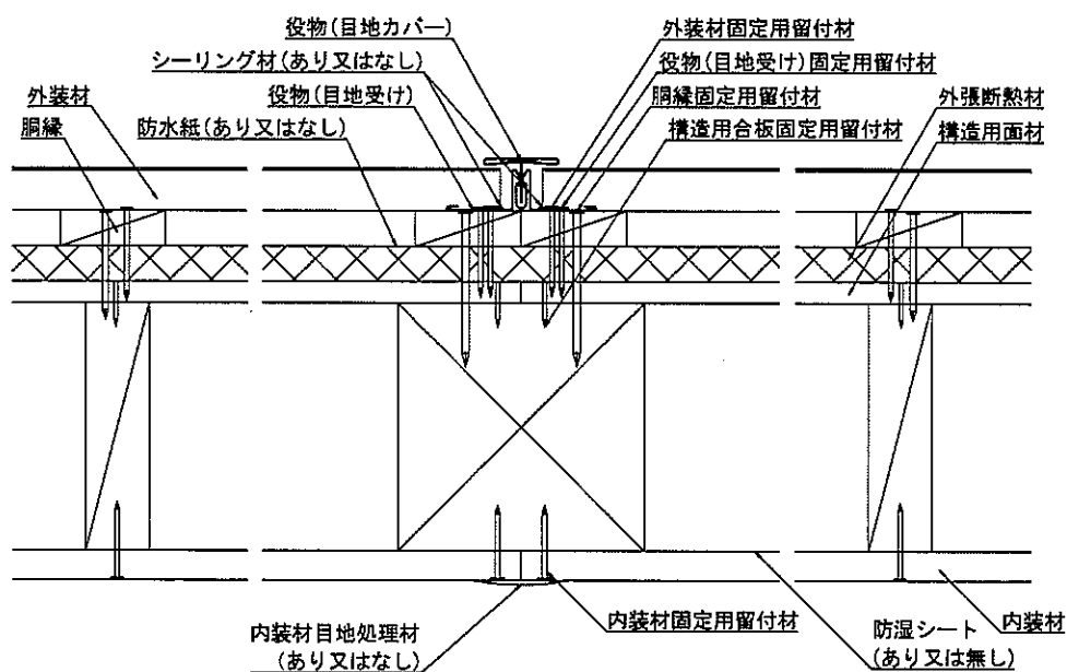
水平断面図
