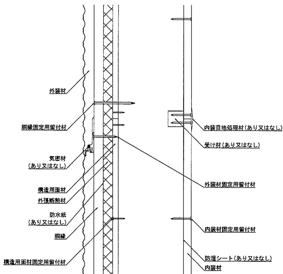
鉛直断面図
