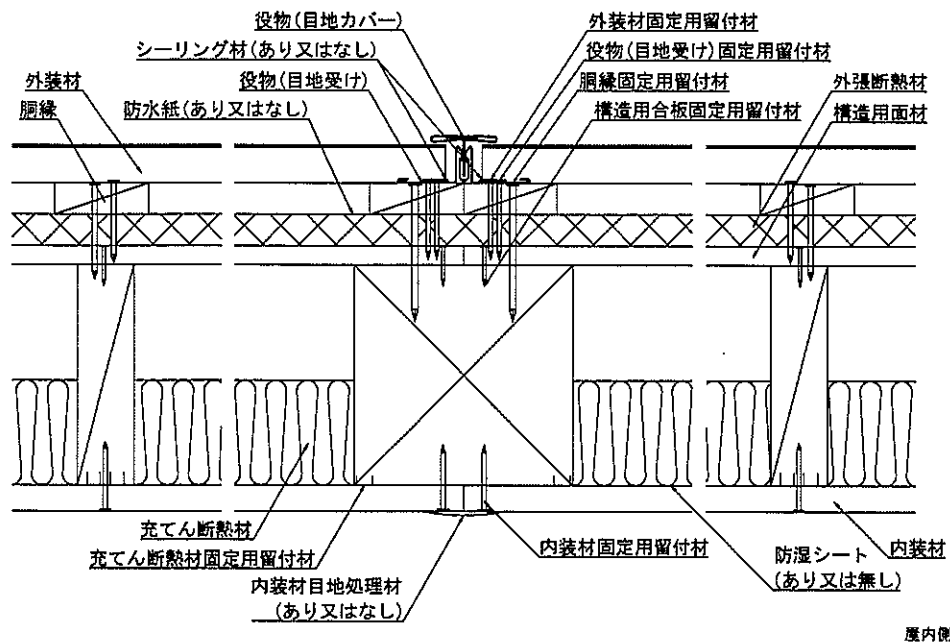
水平断面図
