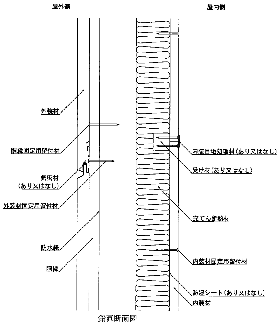
図2 構造説明図
