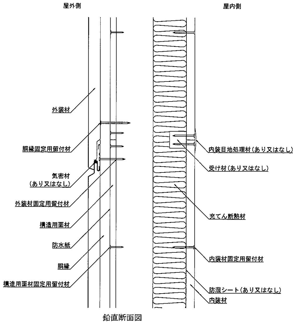
図 2 構造説明図
