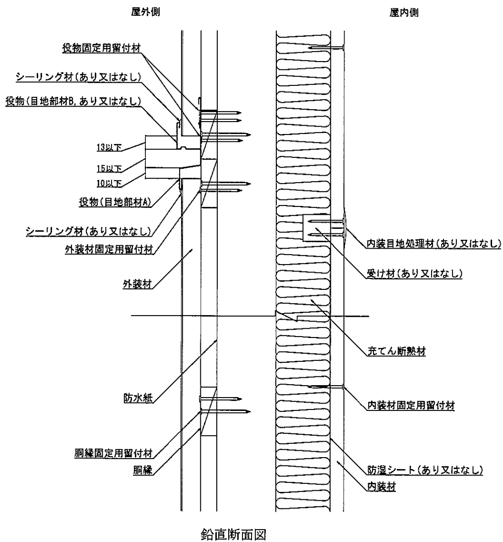
図2 構造説明図
