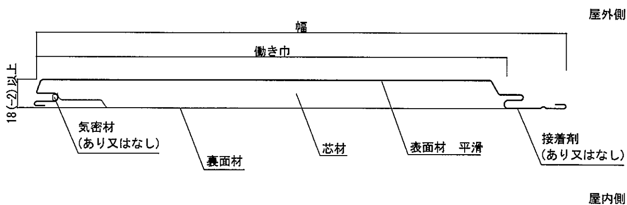
外装材断面
