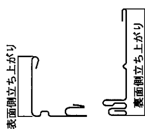
目地部材B(2ピースタイプ)
