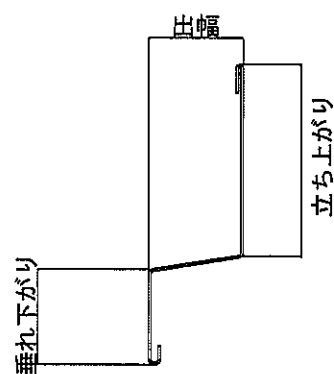
目地部材A 断面図(例)
