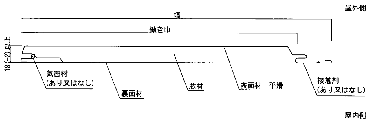
外装材断面
