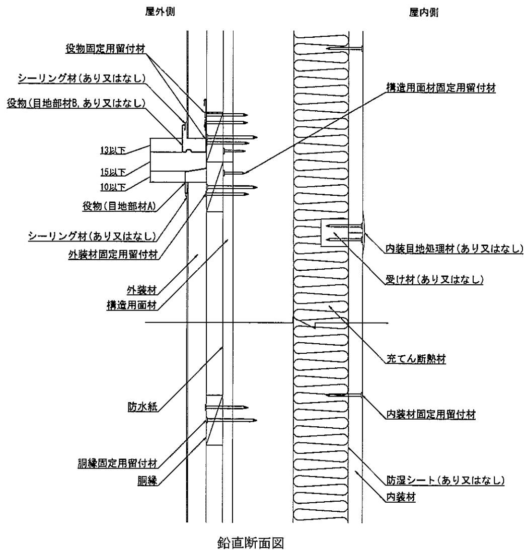
図2 構造説明図
