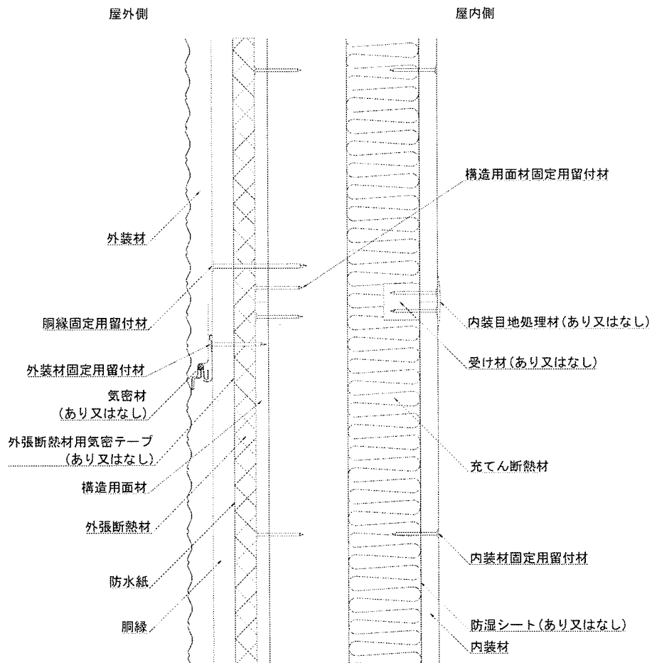
鉛直断面詳細図 図 2 構造説明図(充てん断熱材あり)
