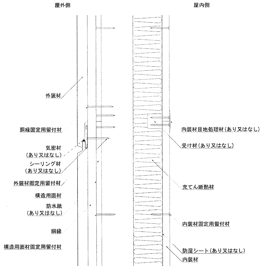
図2 構造説明図
