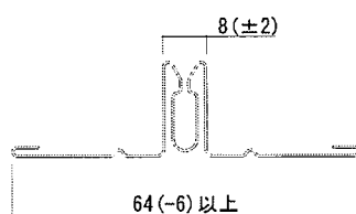
目地受け(銅板製)
