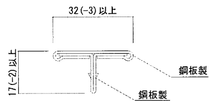
目地カバー(2ピースタイプ)
