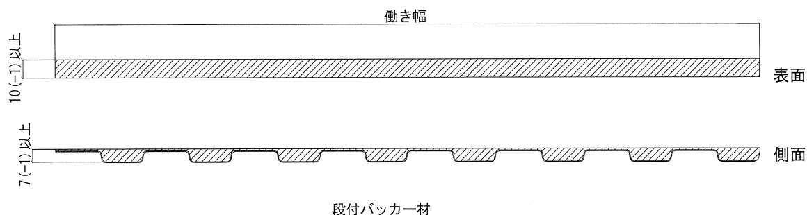
目地部材B 断面図(例)
