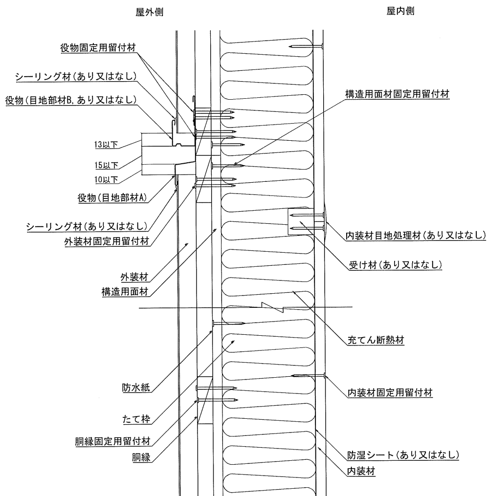
鉛直断面図
