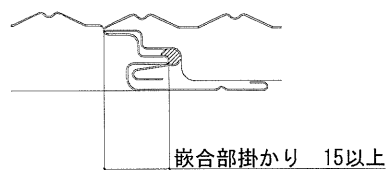
嵌合部詳細(例)
