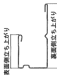
目地部材B 断面図(例)
