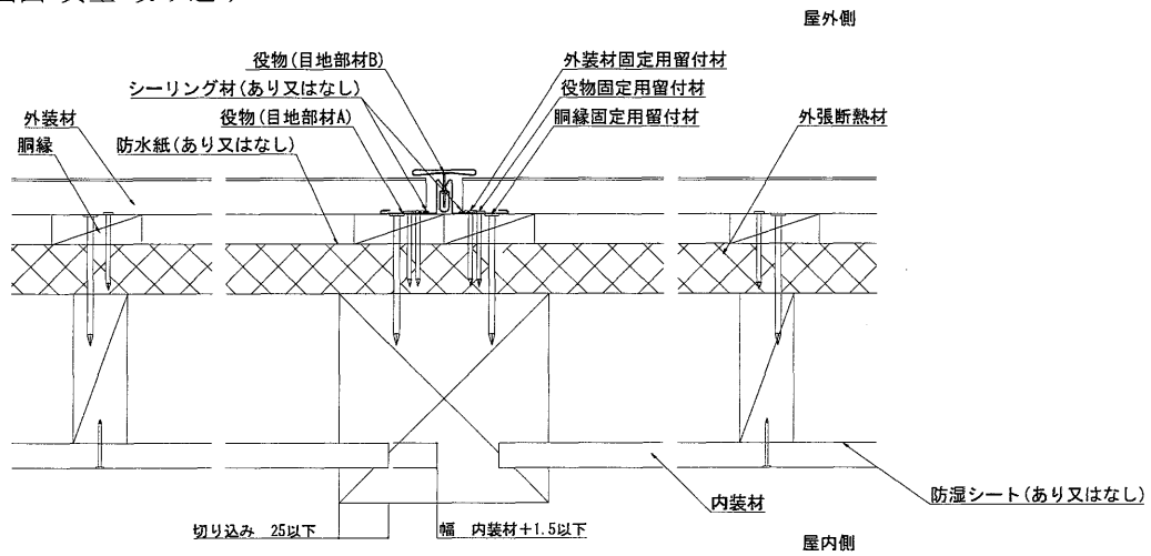
<水平断面図-真壁-受け材>
