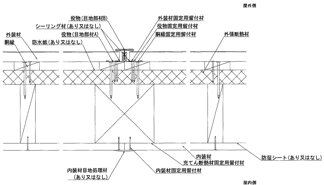
<水平断面図-大壁>
