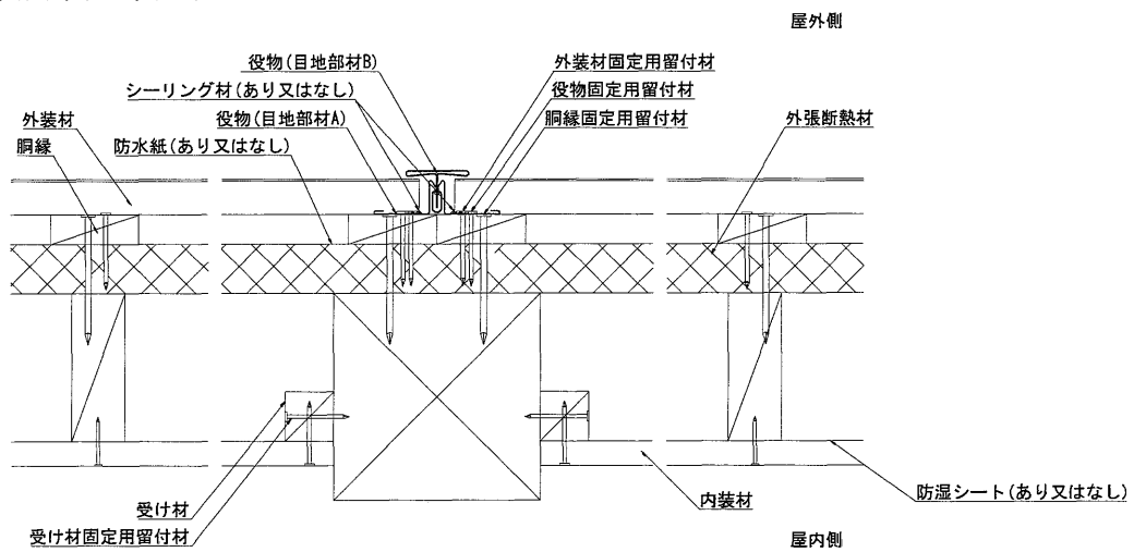
<水平断面図-大壁>
