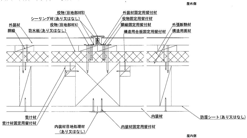
<水平断面図 面材：真壁、内装材：大壁>
