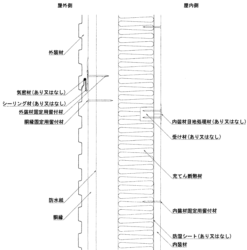
水平断面図
