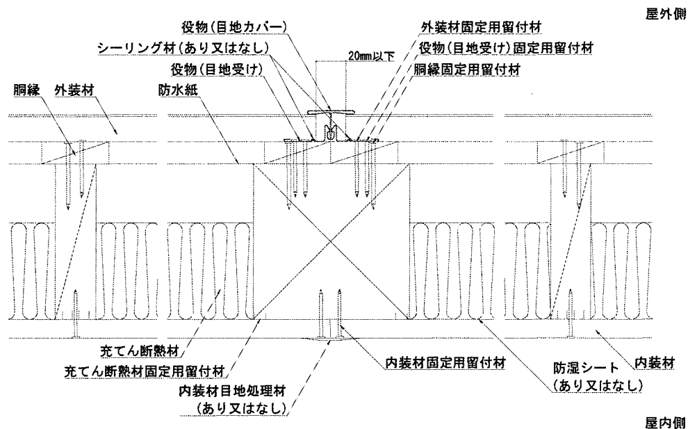
水平断面図
