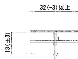
目地カバー (鋼板製) 2ピースタイプ
