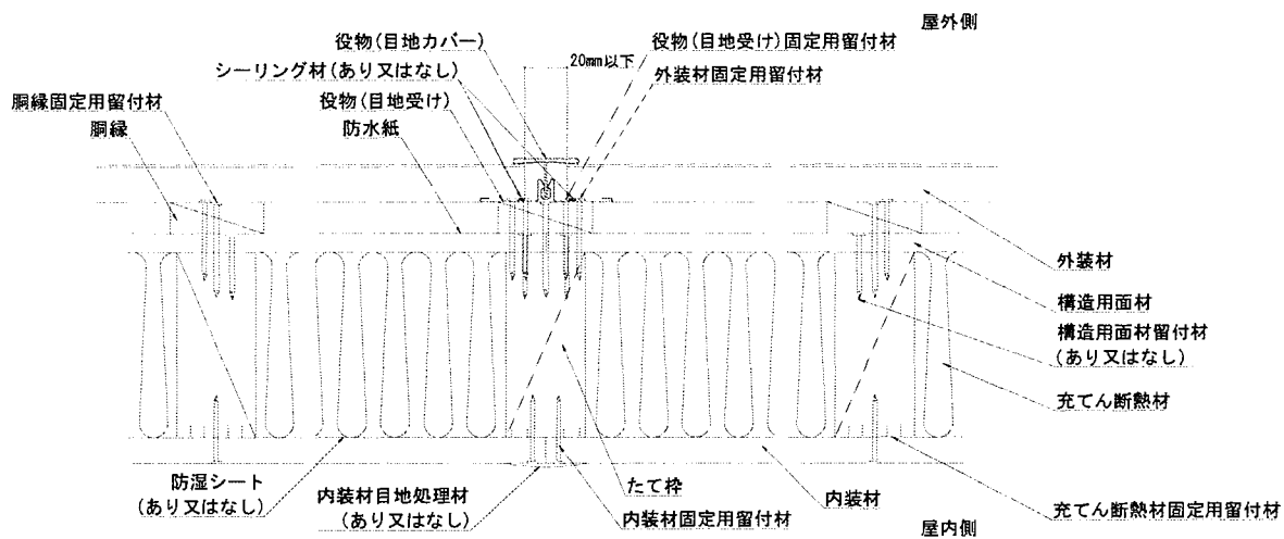
水平断面図
