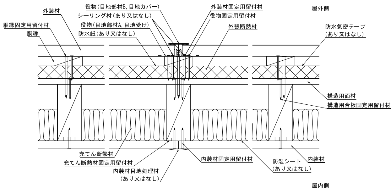
水平断面図
