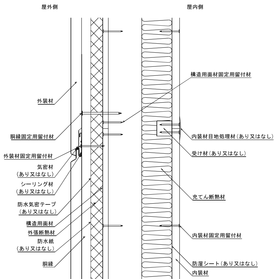
鉛直断面図
