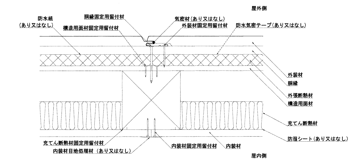
図3 構造説明図(構造用面材あり、充てん断熱材あり)
