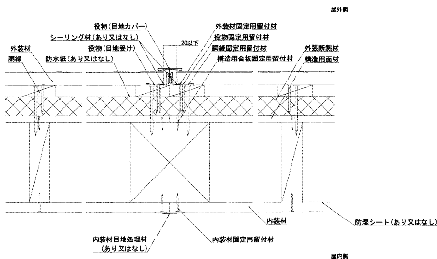
図 3 構造説明図(構造用面材あり、充てん断熱材なし)
