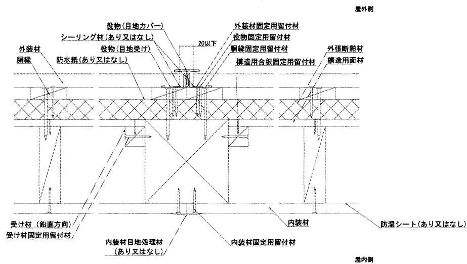
図 2 構造説明図(構造用面材あり、充てん断熱材なし)
