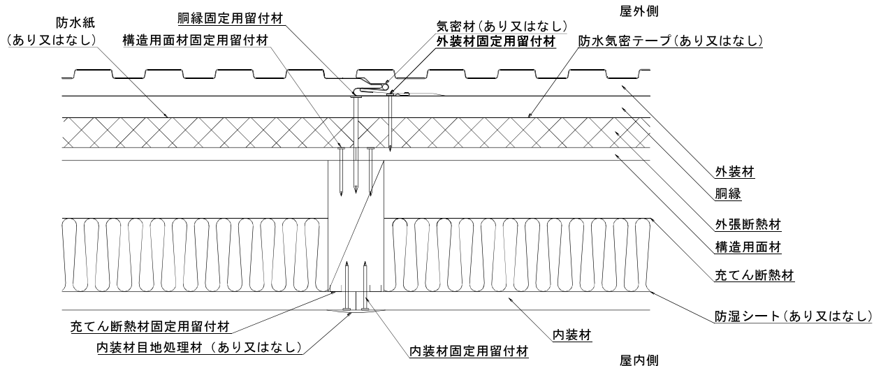
水平断面図
