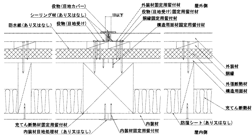
図 3 構造説明図(構造用面材あり)
