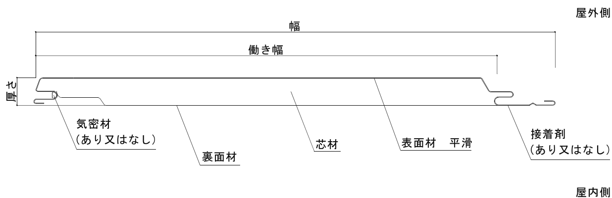
外装材断面
