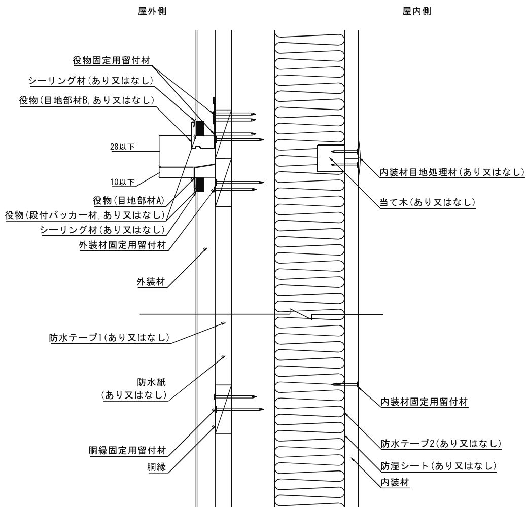
鉛直断面図
