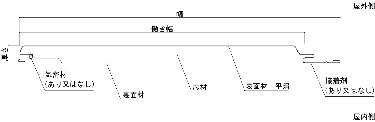
外装材断面
