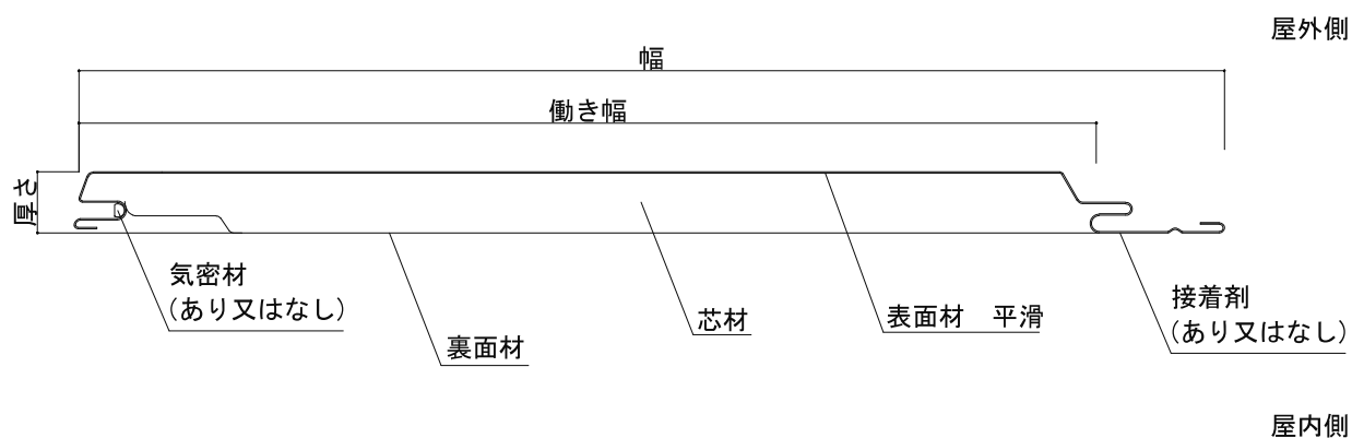
外装材断面
