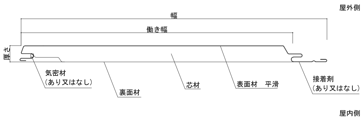
外装材断面
