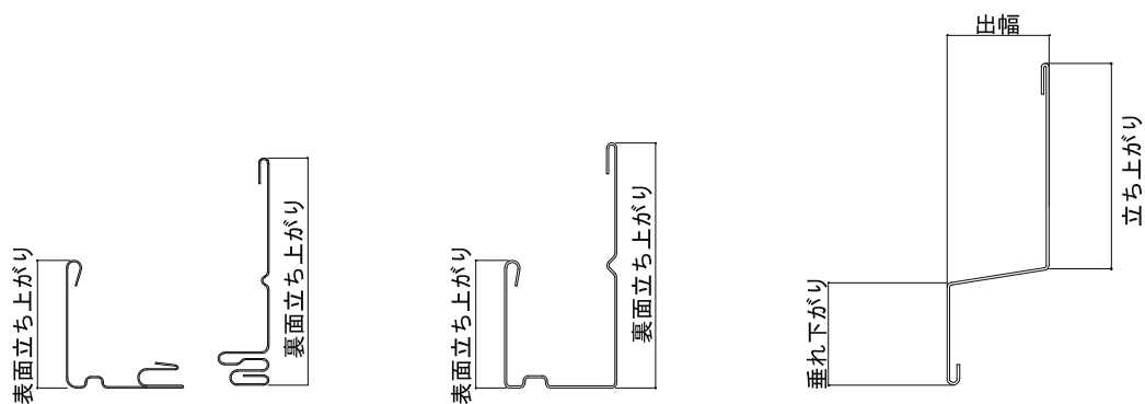
目地部材B(2ピースタイプ) 目地部材B(1ピースタイプ) 目地部材B(カバー) 断面図 例
