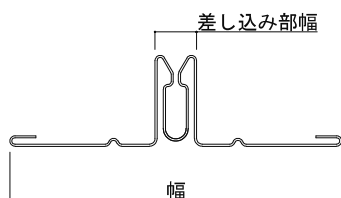
目地部材A(目地受け, 鋼板製)
