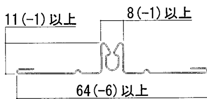
目地受け
