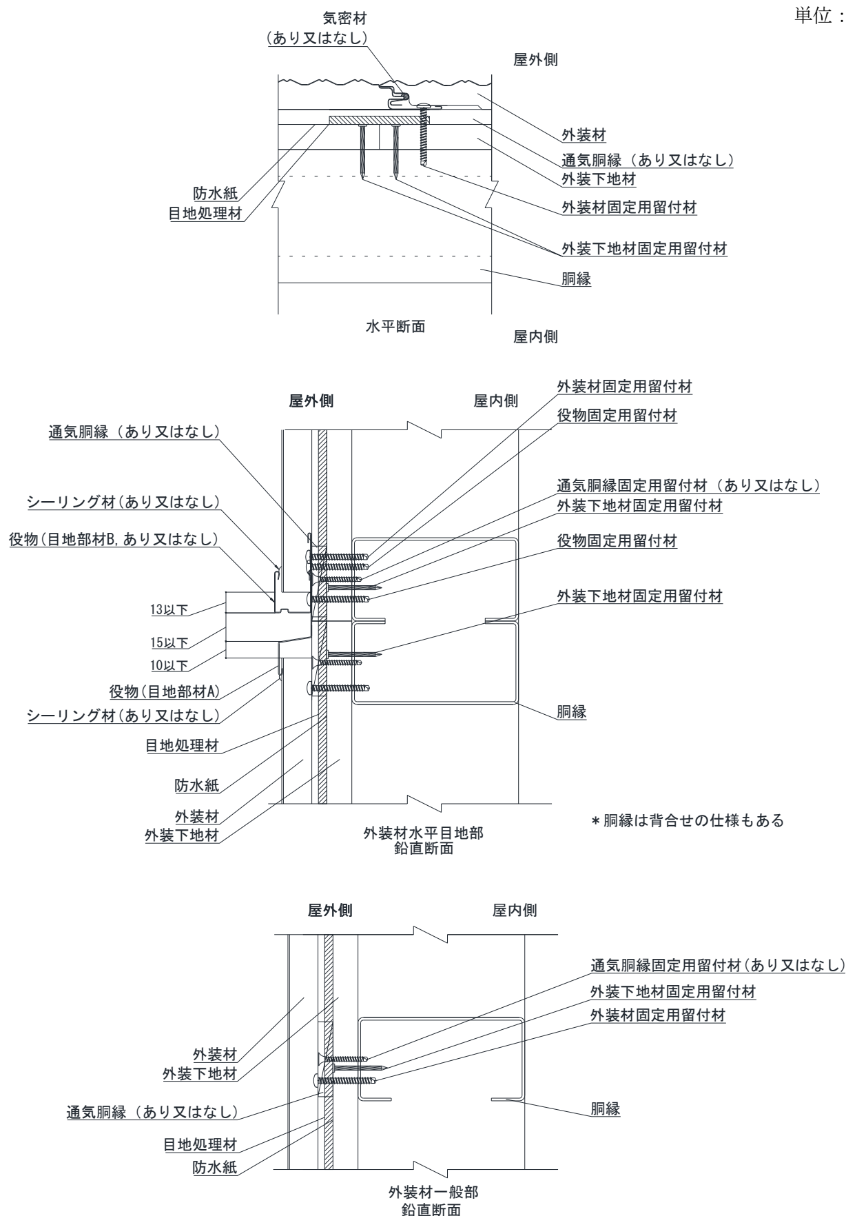
図2 構造説明図 (胴縁が軽量形鋼の場合)
