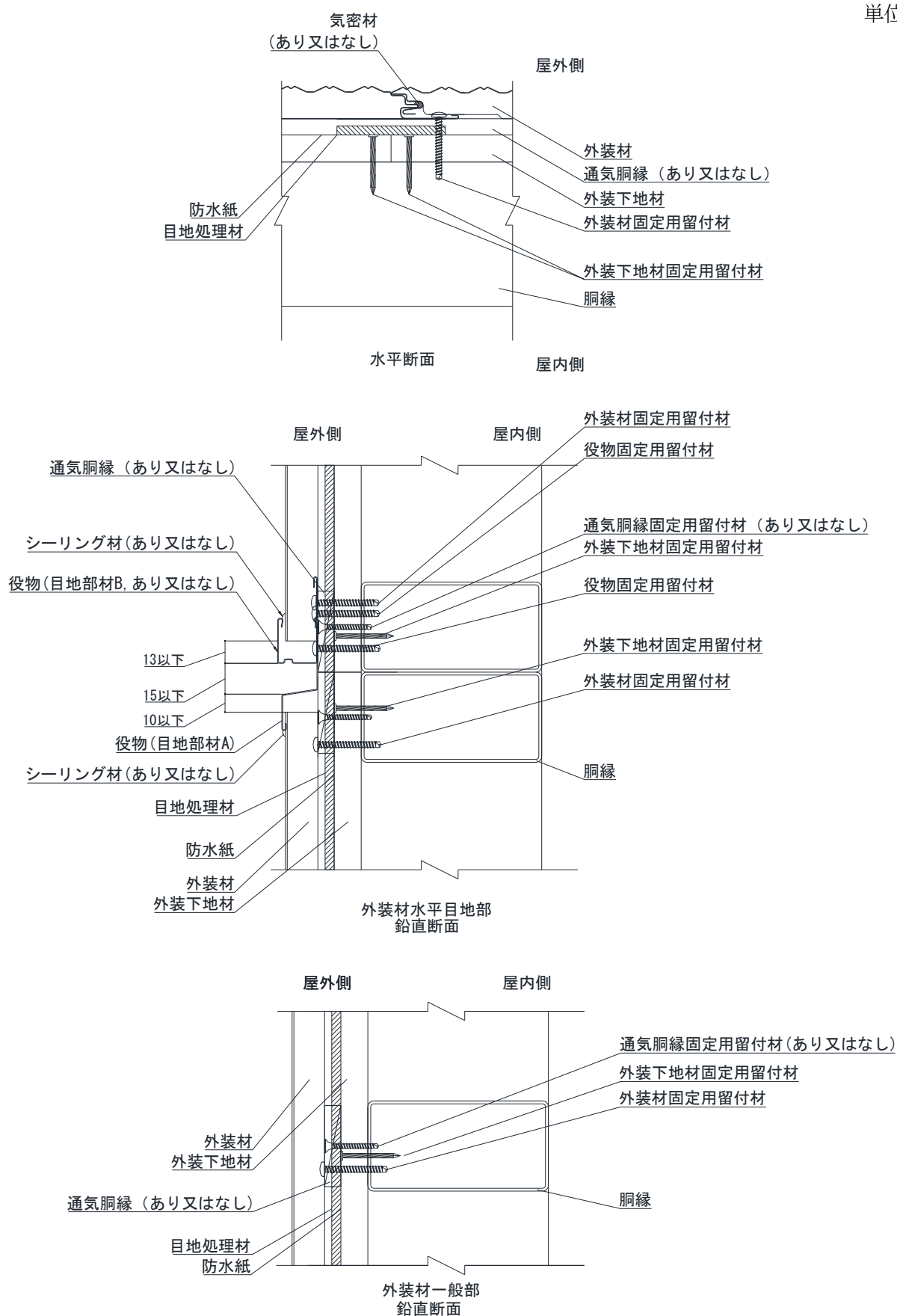
図4 構造説明図 (胴縁が一般構造用角形鋼管の場合)
