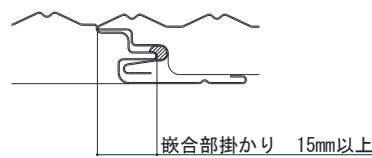
嵌合部詳細
