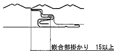
嵌合部詳細(例)
