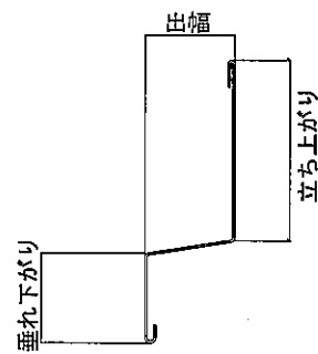
目地部材A 断面図(例)
