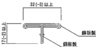
目地部材B(2ピースタイプ)
