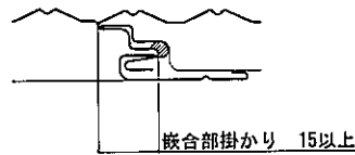
嵌合部詳細(例)
