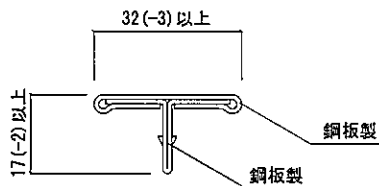
目地部材B(2ピースタイプ)
