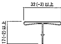
目地部材B(1ピースタイプ)
