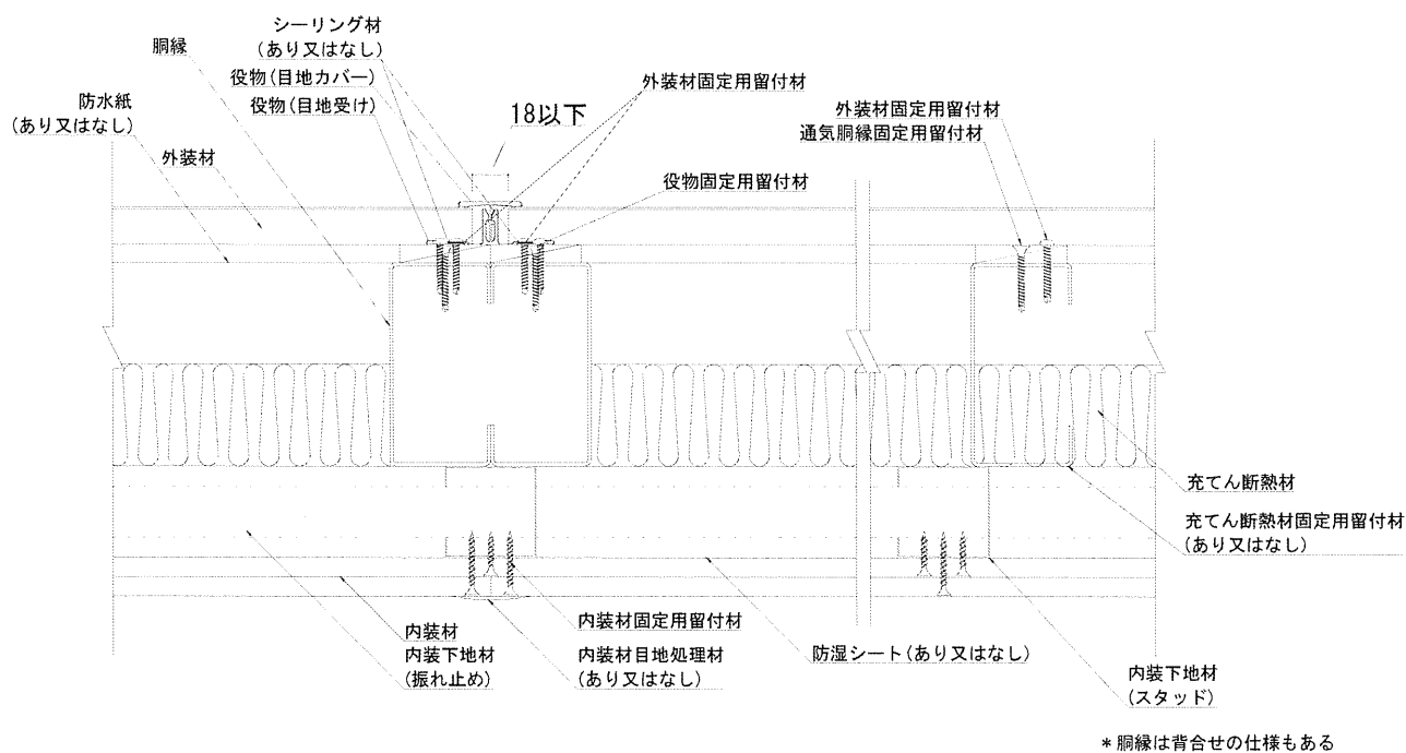
図3 構造説明図 (外装下地材なし／充てん断熱材あり)
