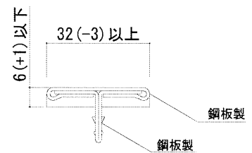
目地部材B(2ピースタイプ)
