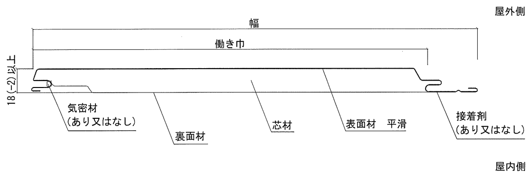
外装材断面
