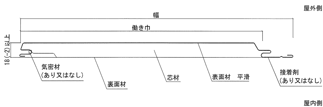
外装材断面
