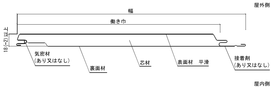
外装材断面
