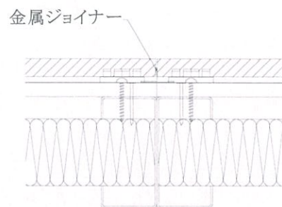
②金属ジョイナー目地
