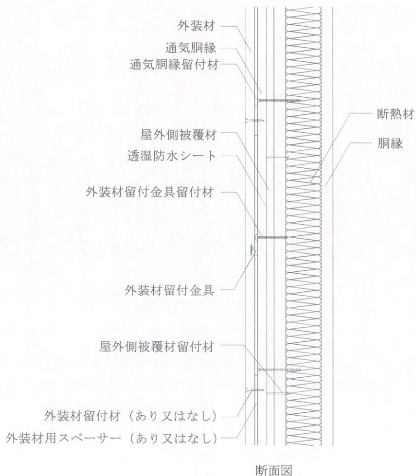
図 4 構造説明図 (通気胴縁仕様)
