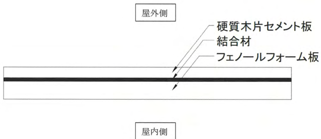
屋外側被覆材(上張り)
