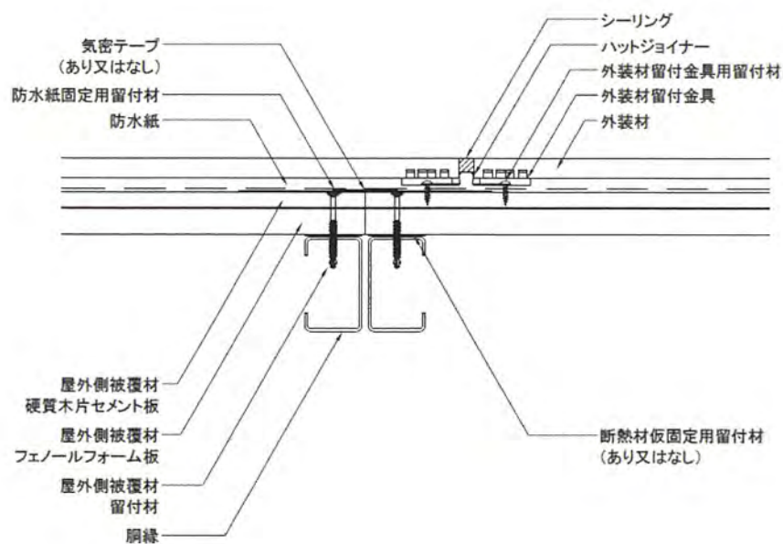
水平断面詳細図
