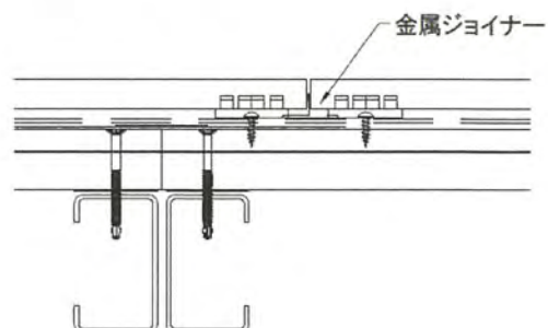
②金属ジョイナー目地
