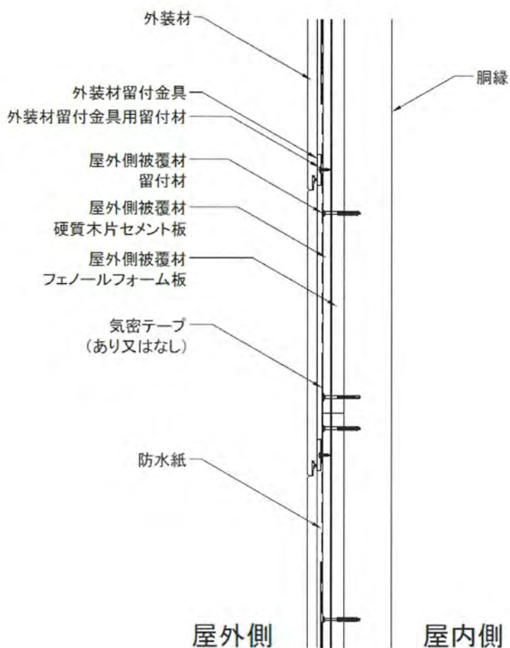
水平断面詳細図
