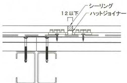
①ハット型ジョイナー+シーリング目地
