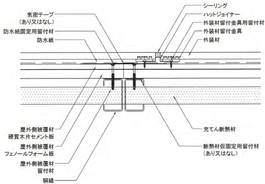
水平断面詳細図
