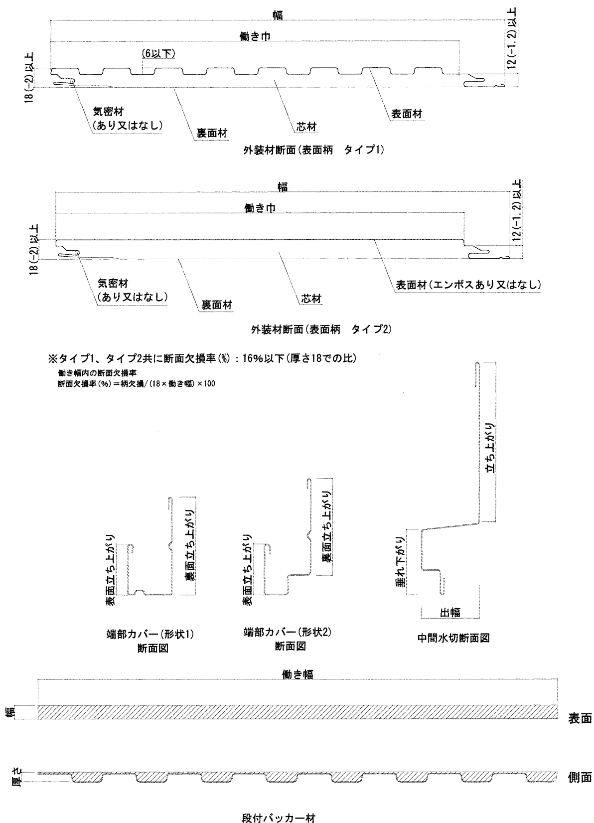
図3 構造説明図
