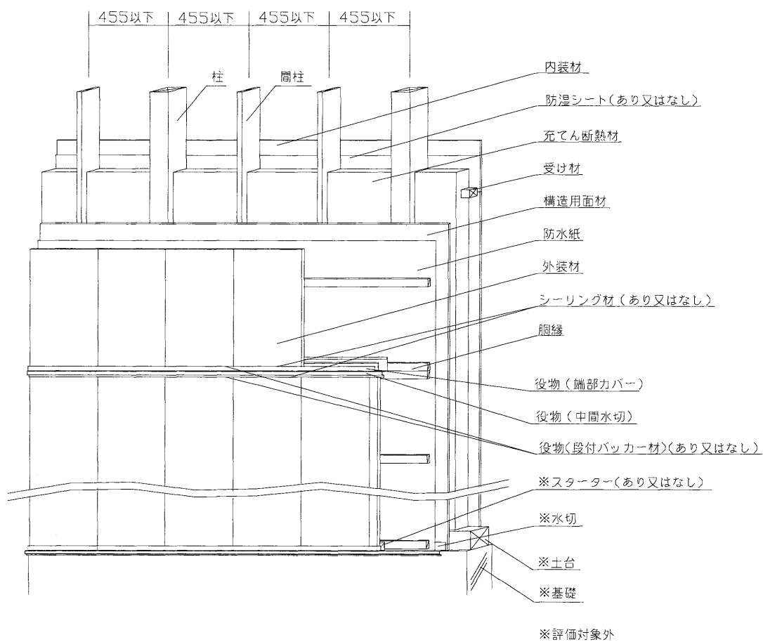
透視図
