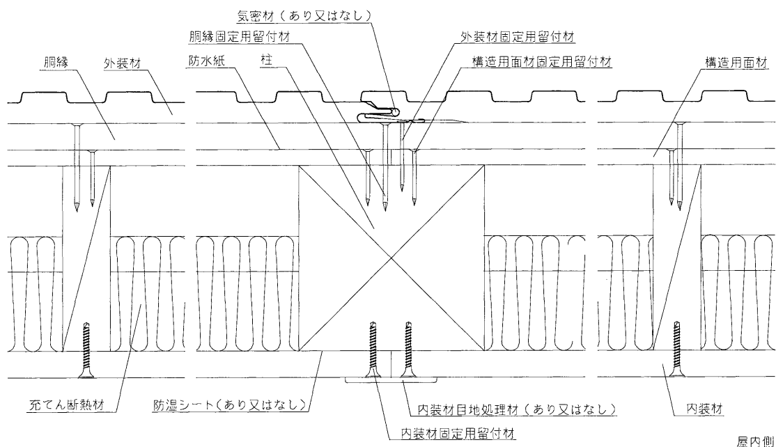
水平断面図
