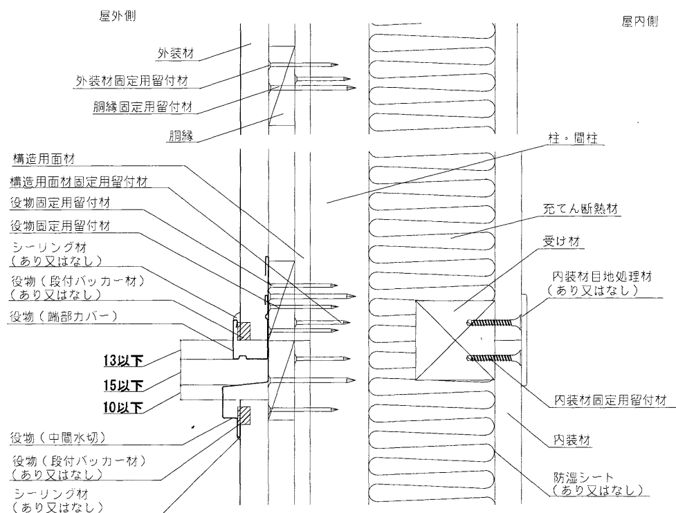
鉛直断面図
