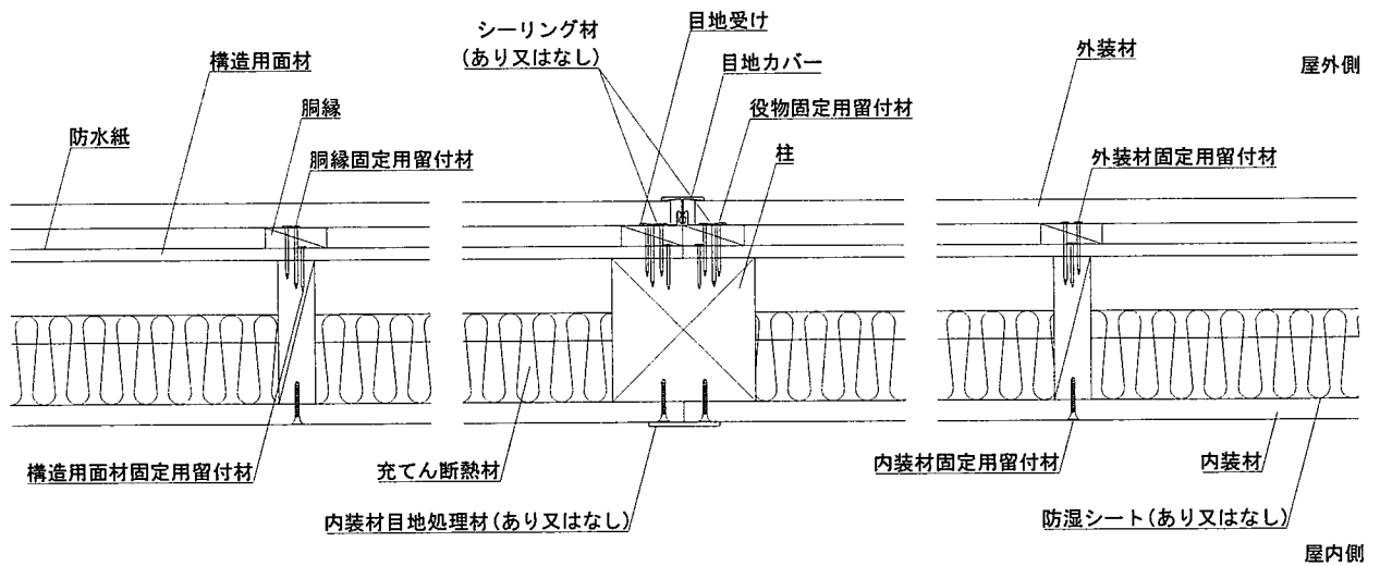
水平断面図
