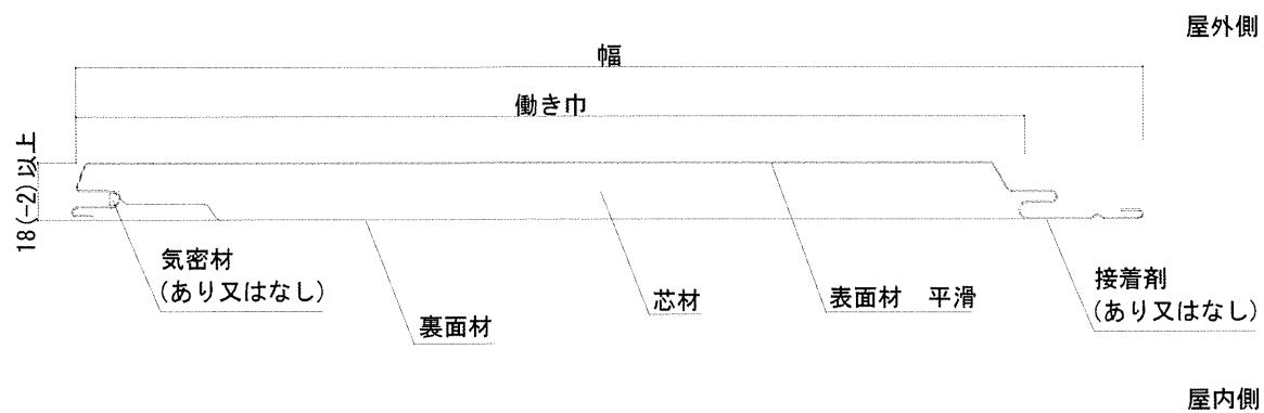
外装材断面
