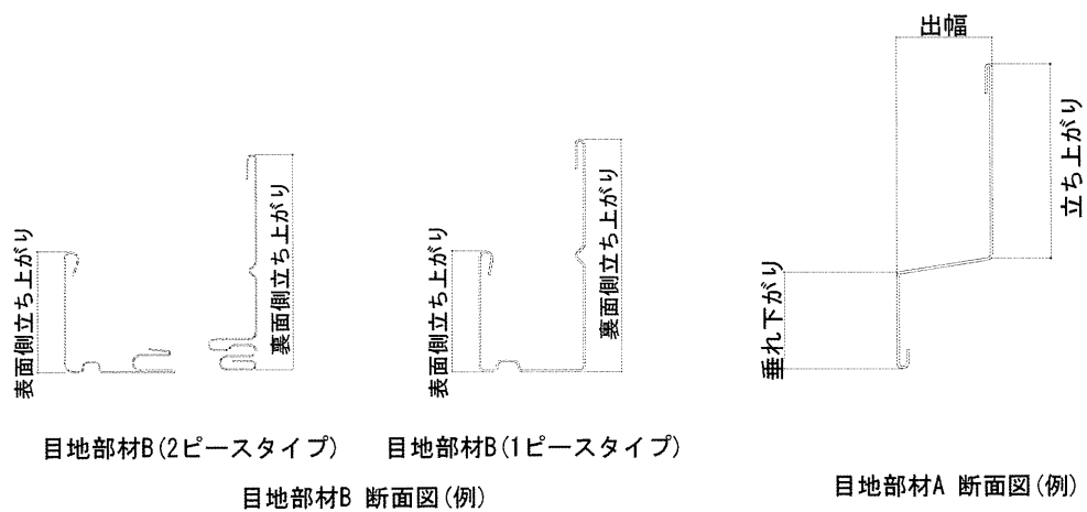
図 3 構造説明図
