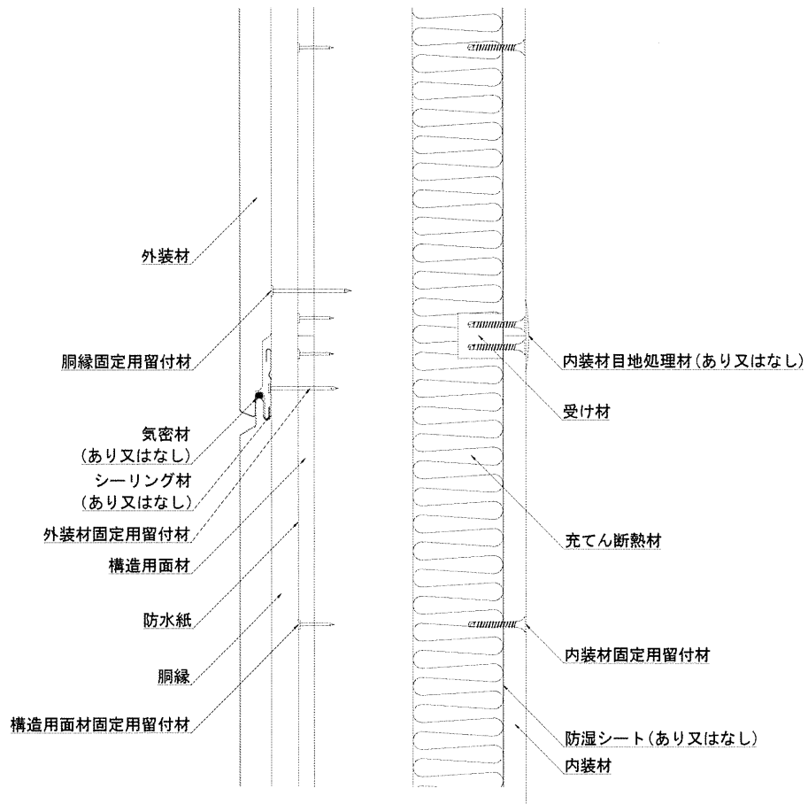
図 2 構造説明図
