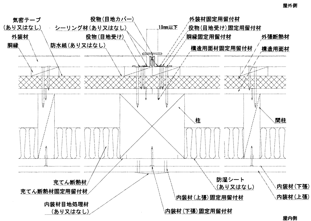
水平断面詳細図
