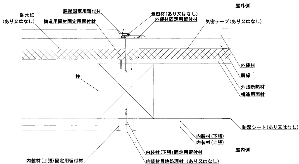
水平断面詳細図
