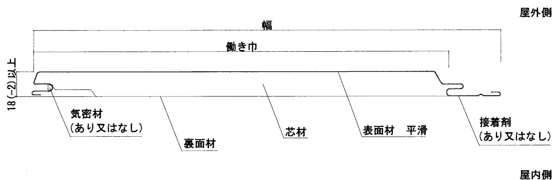
外装材断面
